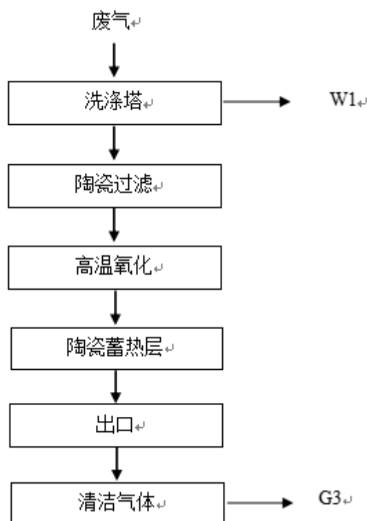
图 4.1-2 切换阀式 RTO 炉废气处理工艺
