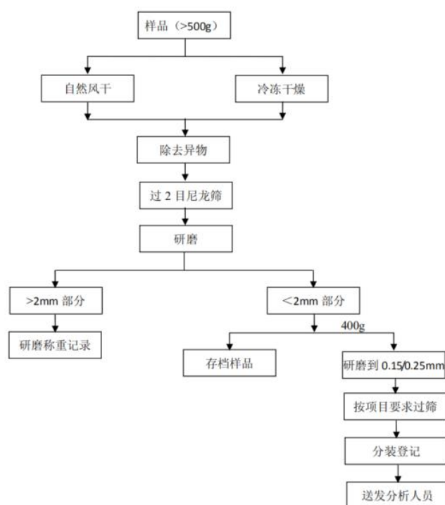
图 7.3-2 土壤样品制样流程图
