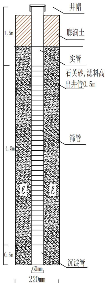
图 7.2-4 地下水采样井结构示意图
