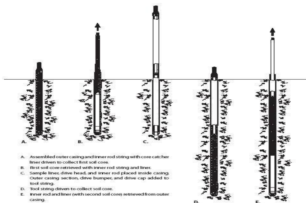
图7.2-3 Geoprobe土壤取样示意图
